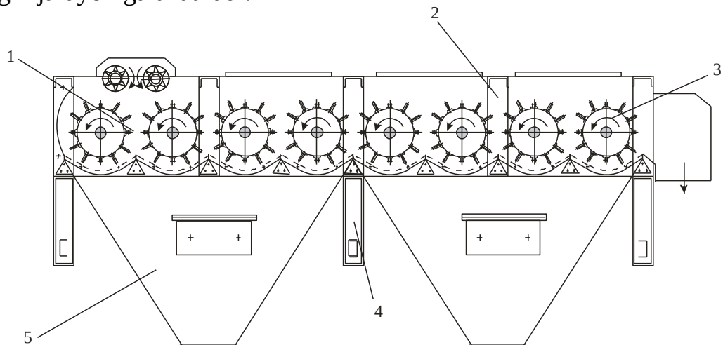
1-rasm. 1XK rusumli mayda iflosliklardan tozalash uskunasi sxemasi
