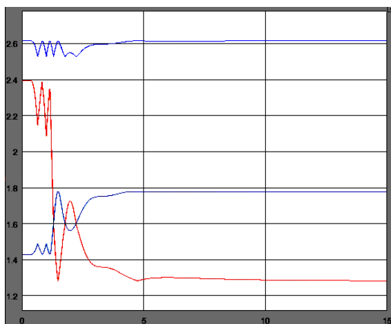
3 - rasm. PID-rostlagich parametrlarining o'zgarish grafigi
