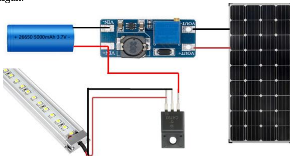
3-rasm. Korxonalardagi ko‘cha chiroqlarini yoritish tizimini avtomatlashtirish sxemasi
