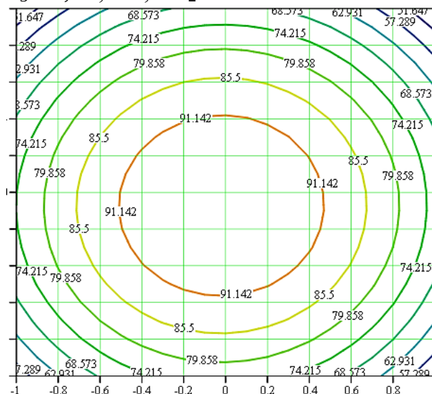
1-rasm. Murakkab tuzilishga ega to'qimaning havo o'tkazuvchanligiga X_1 -xomashyoda paxta tola ulushi, X_3 - ip buramlar soniga bog'liqlik izochizqlari
