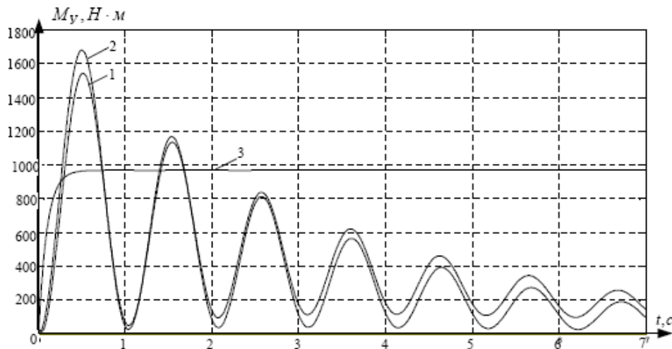
Рис. 2. Графики изменения упругого момента M_y при ступенчатом входном сигнале: 1, 2 – соответственно реальный и идентифицированный графики M_y(t) ; 3 – изменение момента M_y с включением ФР
