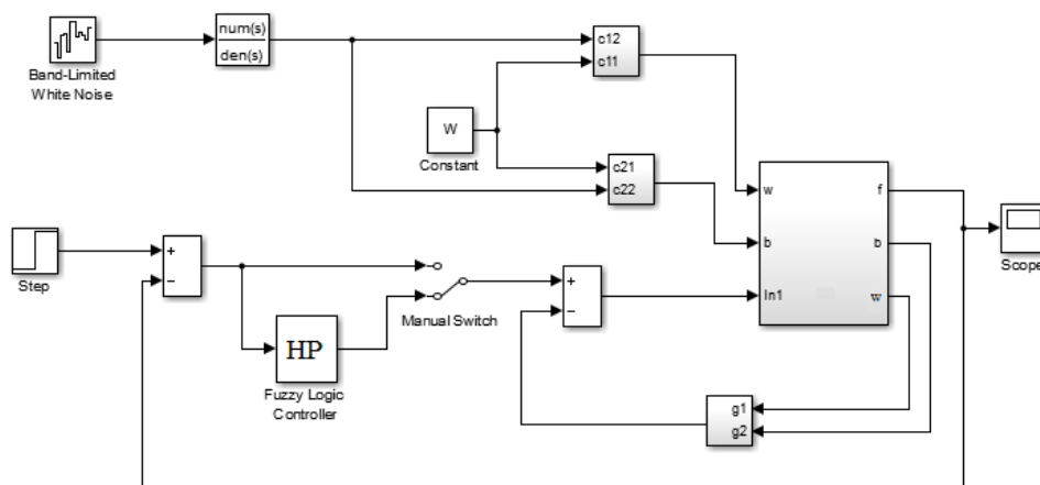
1-rasm. Optimal rostlagich va noqat'iy optimal rostlagichga ega boshqarish tizimlarini tadqiq etish sxemasi.
