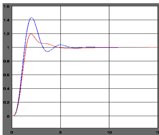
4 - rasm. Klassik va adaptiv PID-rostlagichlarni o'tkinchi jarayonlari tavsiflari
