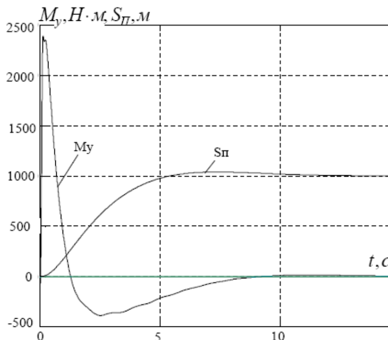
Рис. 4. Графики изменения момента M_y и перемещения рабочего органа S_{II} системы с ПИД-регулятором момента и ФР положения
