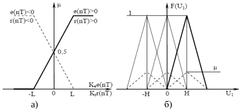
Рис. 3. Функции принадлежности входного (а) и выходного (б) сигналов ФР
