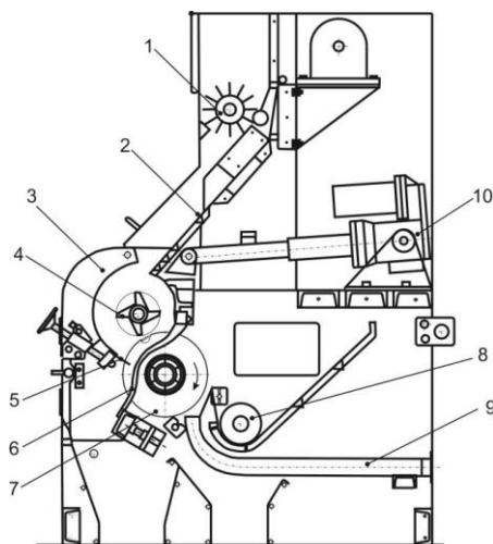
2- rasm. MR-160B-11C rusumli linterining chizmasi.
