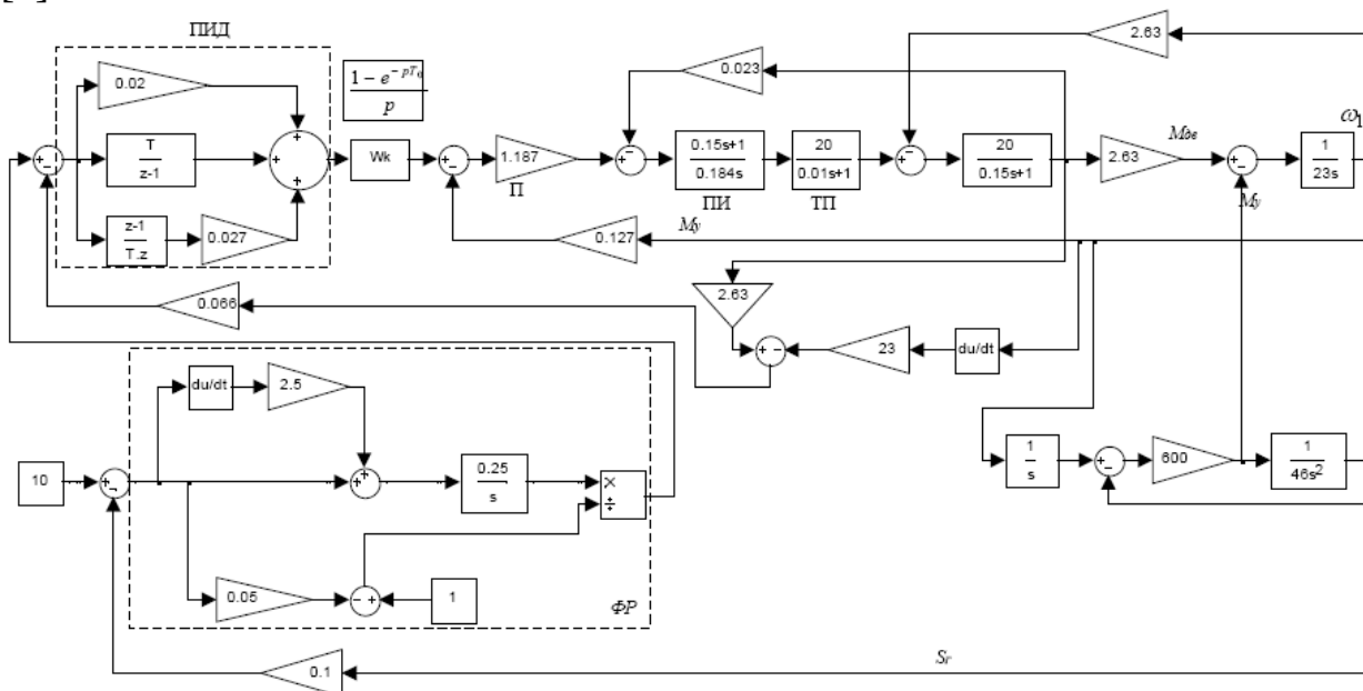
Рис. 1. Simulink – модель четырехконтурной системы управления позиционным электроприводом с упругой механической связью
