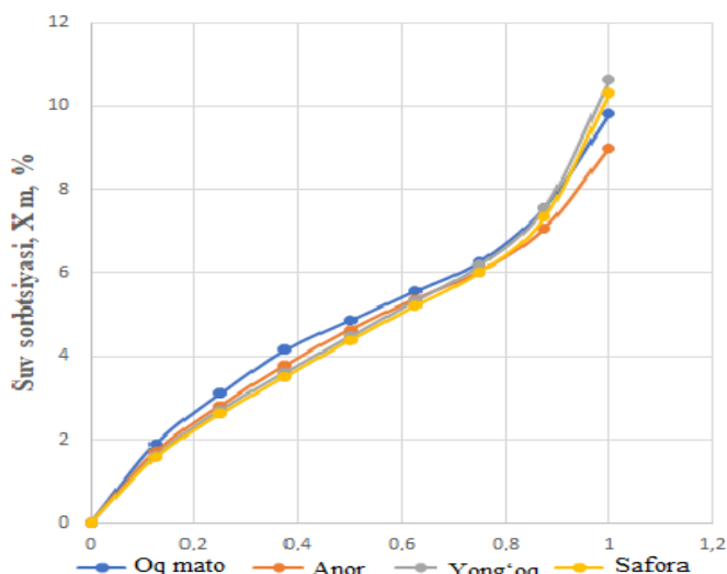
5-rasm. Tabiiy bo'yovchi moddalar bilan bo'yalgan paxta tolali trikotaj matosining sorbsiya xossalari
