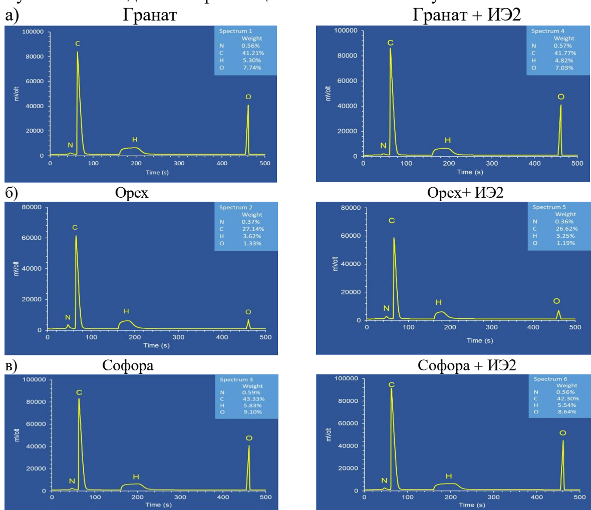
Рис. 2. Элементный анализ природных красителей а- гранатовая кожура, б- околоплодник грецкого ореха, в- софора
