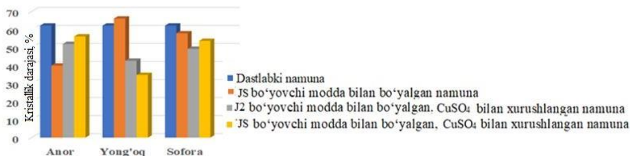
7-rasm. Bo'yalgan matolarning umumiy rentgenostrukturaviy tahlili
