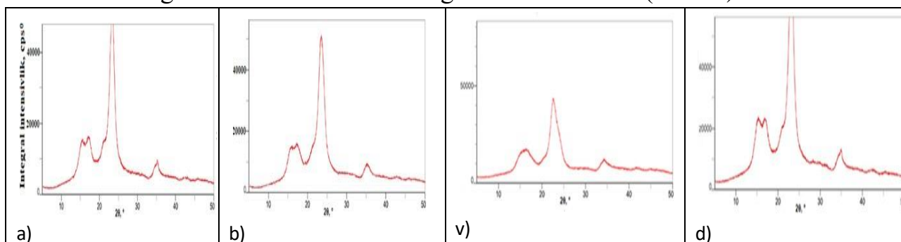
6-rasm. Tabiiy bo'yovchi modda bilan bo'yalgan paxta tolali trikotajning rentgenografik tahlili (anor po'stlog'i). a) Oq mato; b) JS bo'yovchi modda bilan bo'yalgan mato; v) J-2 bo'yovchi modda bilan CuSO_4 tuzi ishtirokida bo'yalgan mato; d) JS bo'yovchi modda bilan CuSO_4 tuzi ishtirokida bo'yalgan mato.
