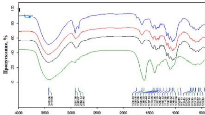
8-rasm. Tabiiy bo'yovchi moddalar bilan bo'yalgan paxta tarkibli trikotaj namunalarining IK-spektr tahlili
