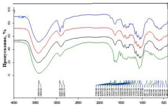
8-rasm. Tabiiy bo'yovchi moddalar bilan bo'yalgan paxta tarkibli trikotaj namunalarining IK-spektr tahlili
