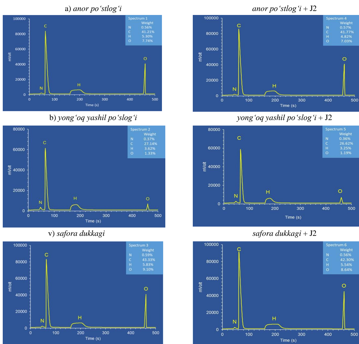
2-rasm. Tabiiy bo'yovchi moddalarning element tahlili
