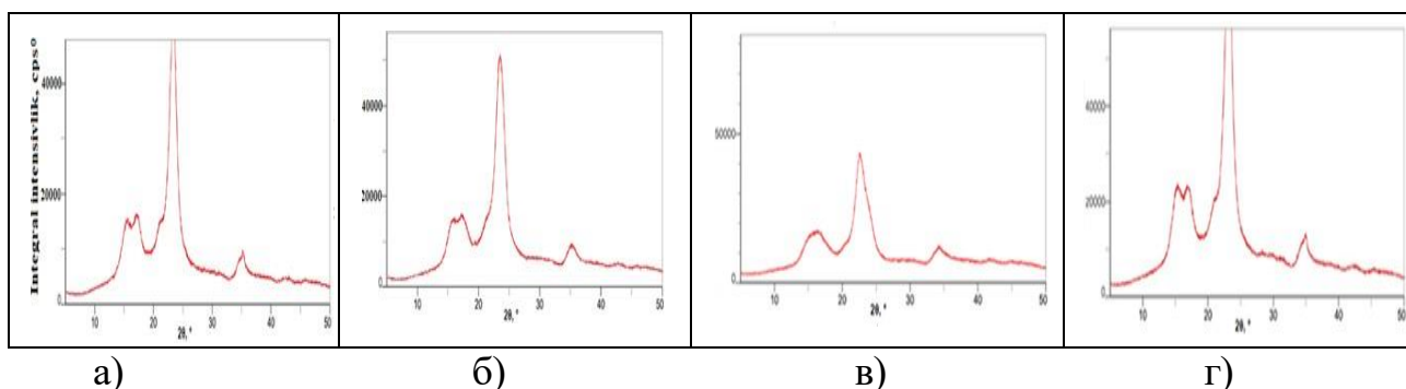
Рис.6. Сравнение степени кристалличности:
